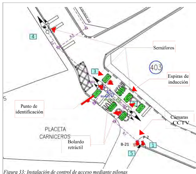
Figura 33: Instalación de control de acceso mediante pilonas
