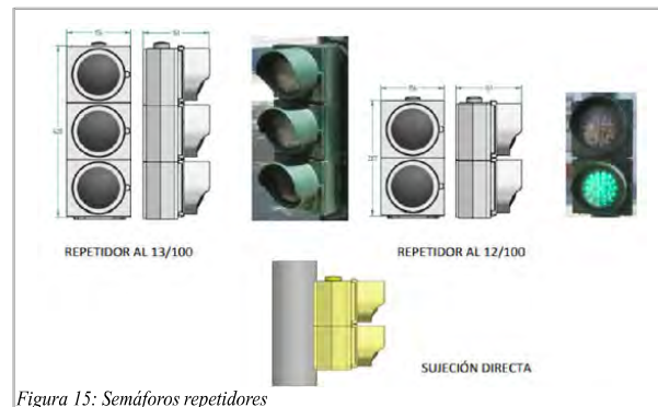
Figura 15: Semáforos repetidores
