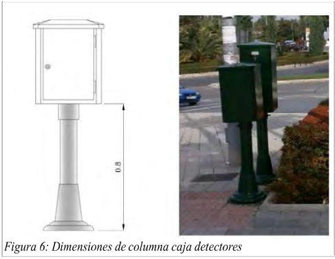
Figura 6: Dimensiones de columna caja detectores
