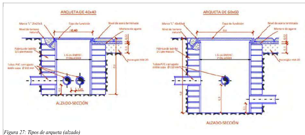
Figura 27: Tipos de arqueta (alzado)
