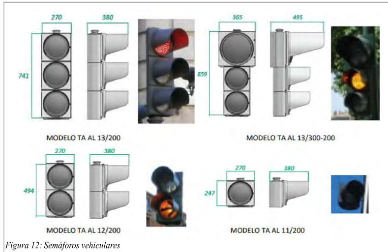
Figura 12: Semáforos vehiculares
