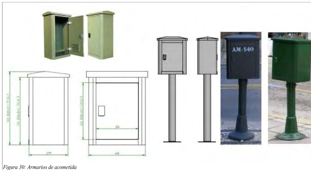
Figura 30: Armarios de acometida
