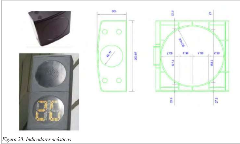
Figura 20: Indicadores acústicos
