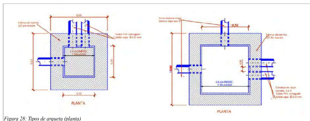
Figura 28: Tipos de arqueta (planta)
