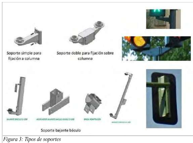
Figura 3: Tipos de soportes
