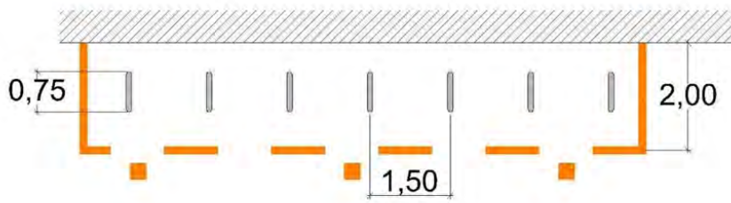
RESERVA DE MOTOS CON HORQUILLAS DELIMITADORAS
