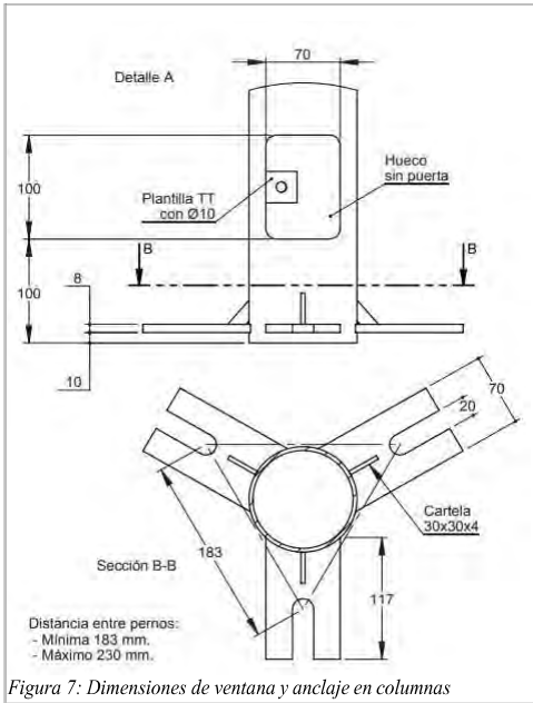
Figura 7: Dimensiones de ventana y anclaje en columnas
