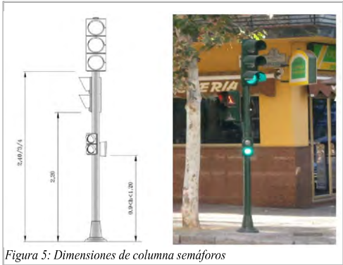
Figura 5: Dimensiones de columna semáforos
