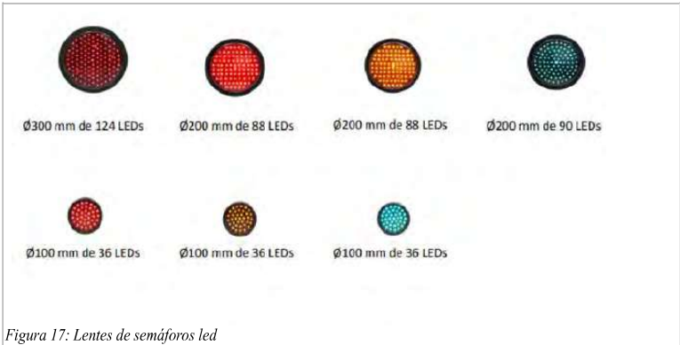
Figura 17: Lentes de semáforos led
